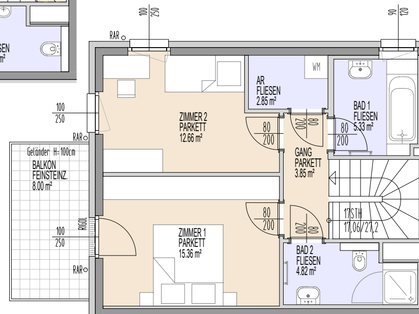
OBERGESCHOSS
