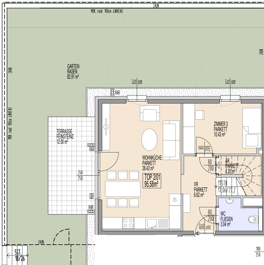
ERDGESCHOSS
